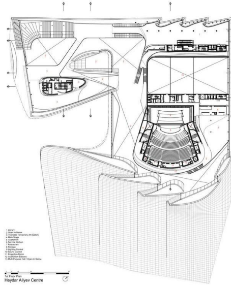
Resim 5: 1. Kat Planı.
