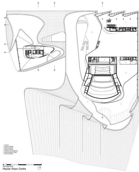
Resim 7: 3. Kat Planı.
