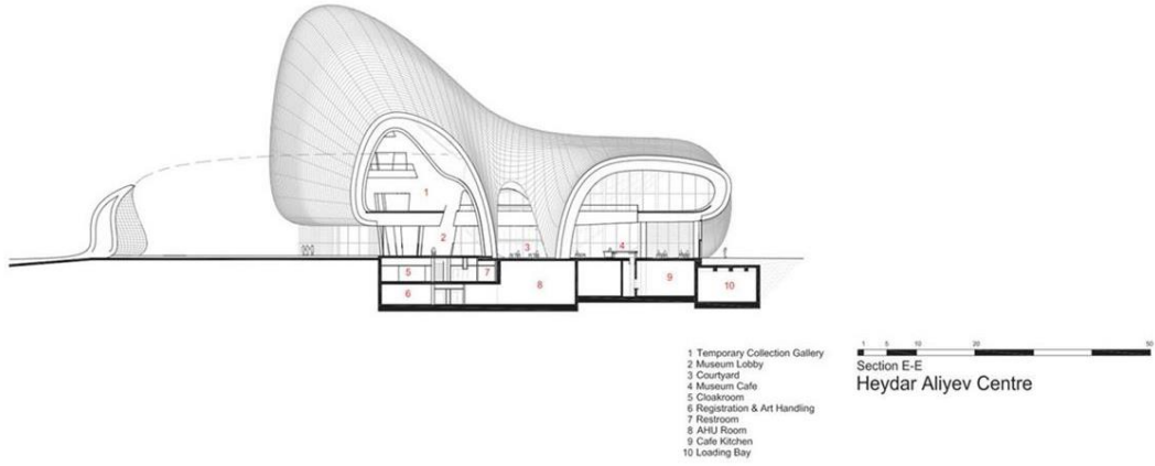
Resim 15: Kesit 2.
