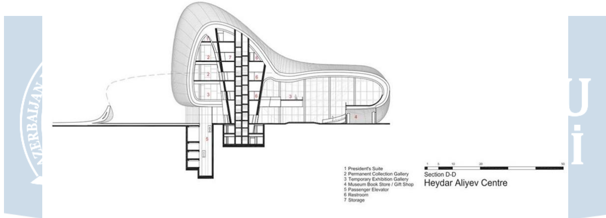
Resim 16: Kesit 3.
