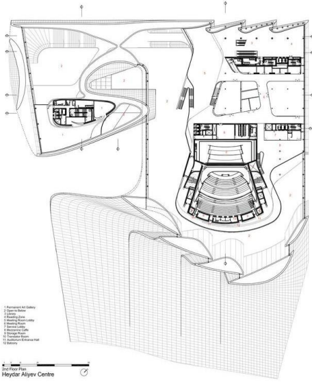
Resim 6: 2. Kat Planı.
