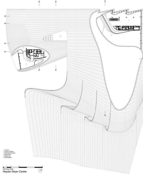
Resim 9: 5. Kat Planı.
