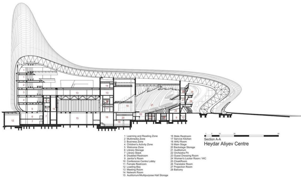
Resim 17: Kesit 4.
