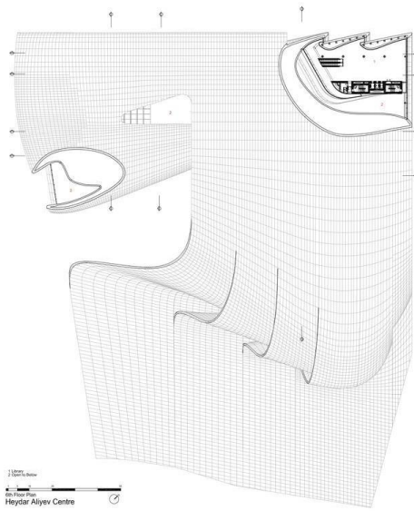
Resim 10: 6. Kat Planı.
