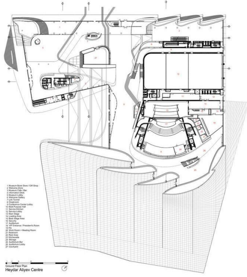
Resim 4: Zemin Kat Planı.
