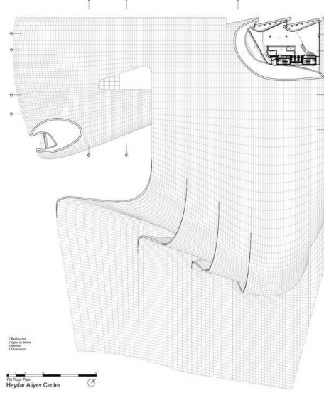
Resim 11: 7. Kat Planı.
