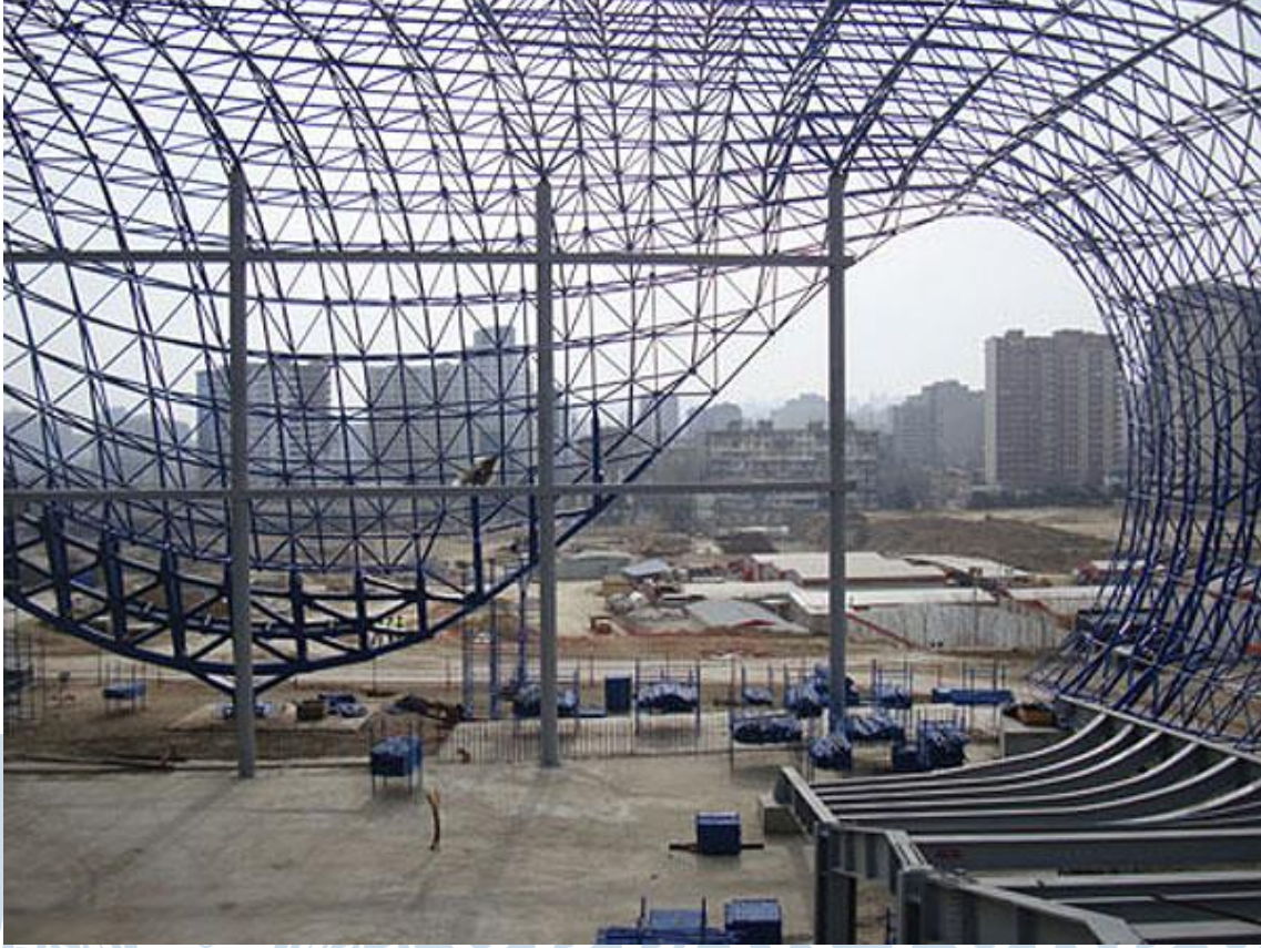
Resim 20: Haydar Aliyev Kültür Merkezi Yapım Aşamaları.
